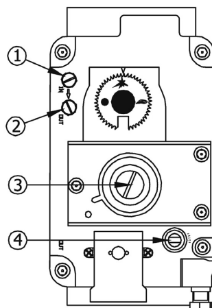
VALVULA SIT 820 NOVA
